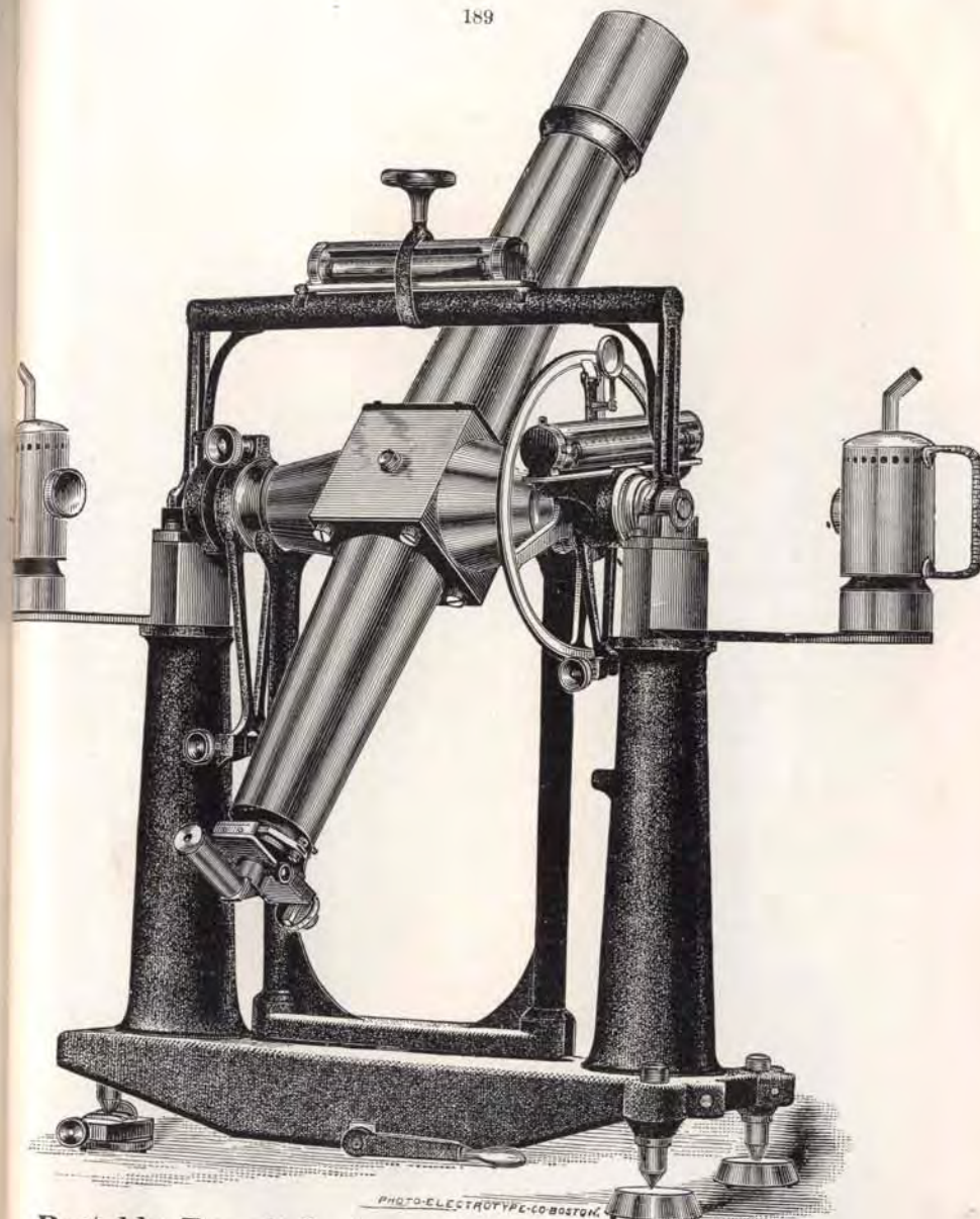
Portable Transit Instrument for Latitude Observations.
