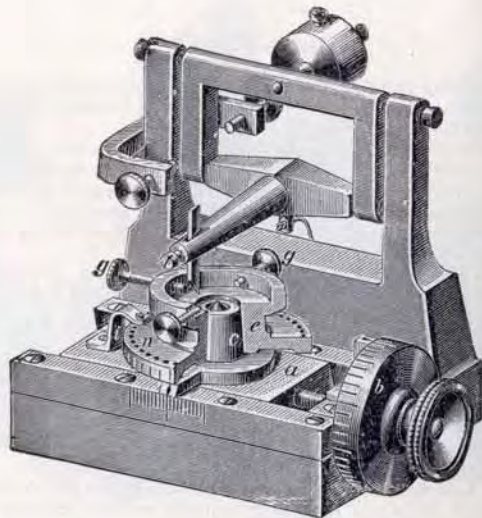
The Longitudinal Dividing Engine.
